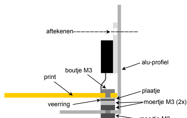
Fig 5: Bevestiging van het aluminium profiel op de print
