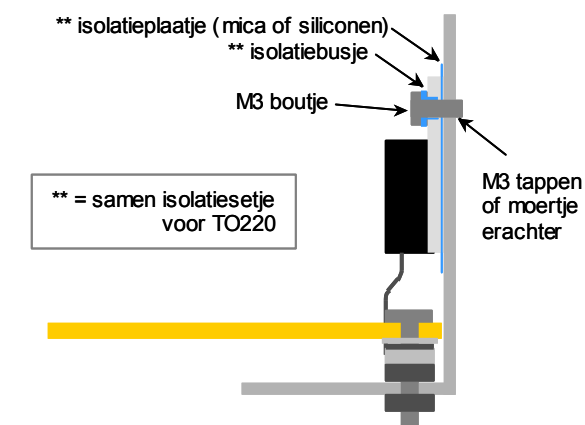
Fig 6: Montage componenten met isolatiesetje
