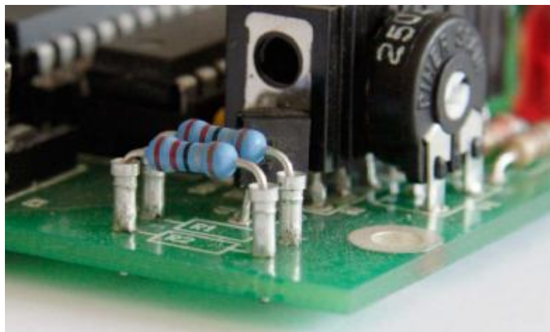
Foto 2: R1/R2 als uitneembare weerstanden in SIL-busjes
