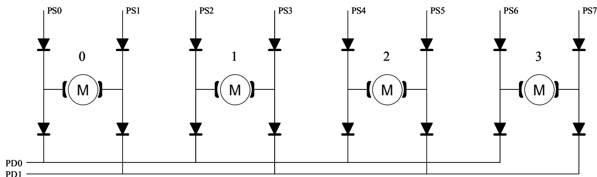
Fig 5: Aansluiten van wisselmotoren op de PM32
