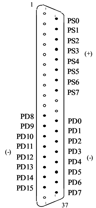
Fig 4: Pinbezetting van K3
