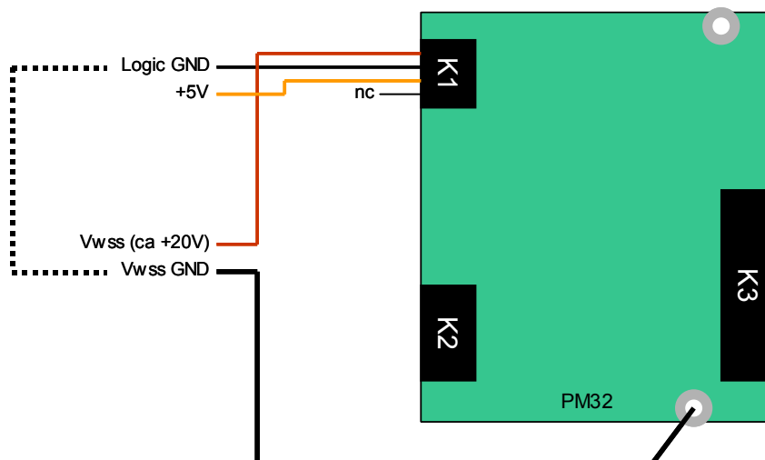
Fig 1: Aansluiten voedingsspanningen
