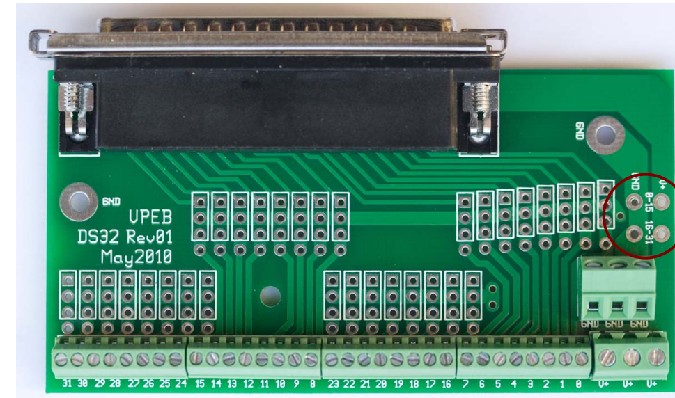
Fig 4. Plaats om de voeding voor de transistoren aan te sluiten
