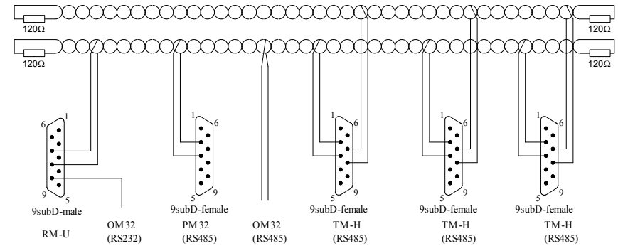
Fig.5: Koppelen van modules via een RS485 netwerk
