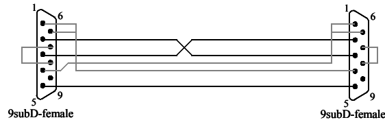
Fig 2: Nulmodemkabel
