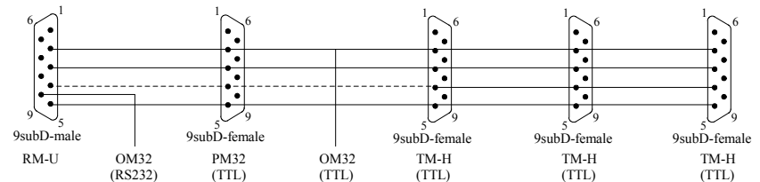
Fig 3: Koppelen van modules met TTL
