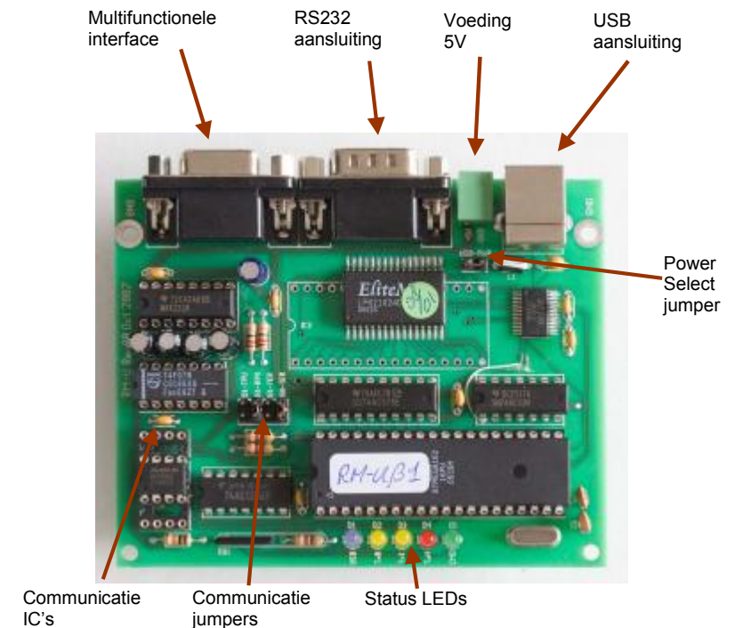
Fig 1: Overzicht van de RM-U
