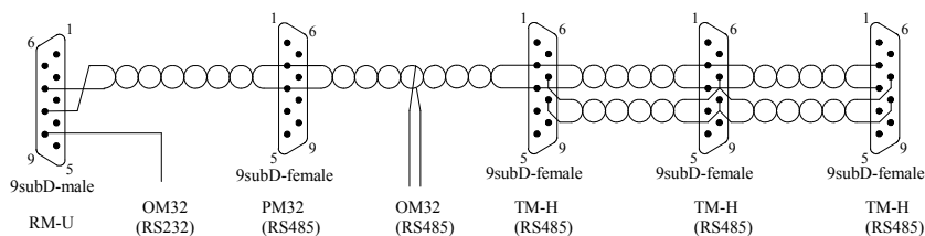
Fig 4: Koppelen van modules met RS485
