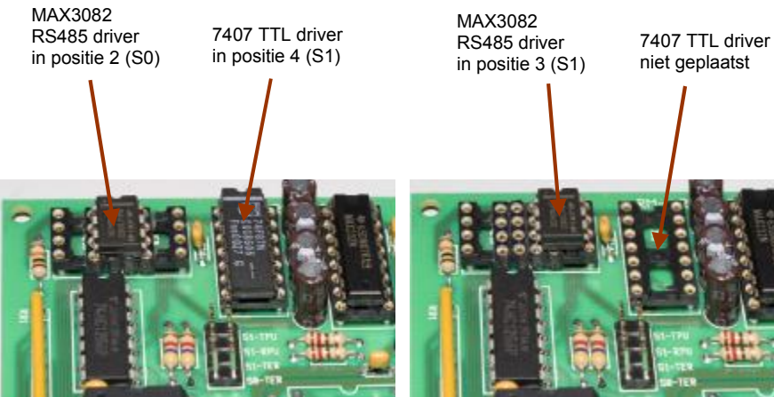
Fig 6: Positie van de communicatie-drivers op de RM-U
