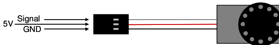
Fig 5: Aansluitingen servo
