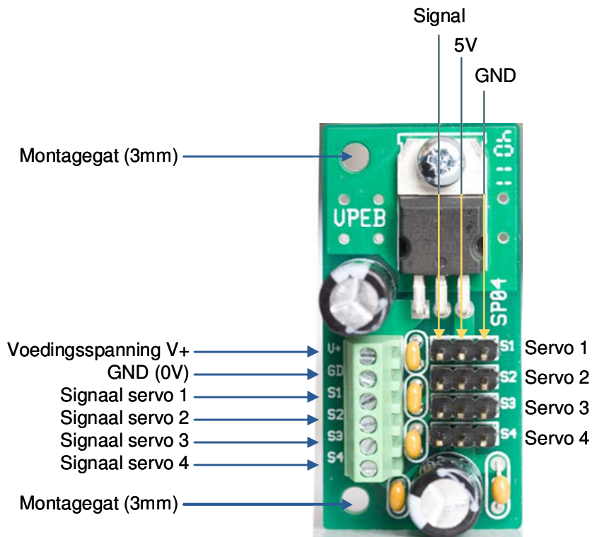
Fig 2: SPO4 overzicht aansluitingen en functies
