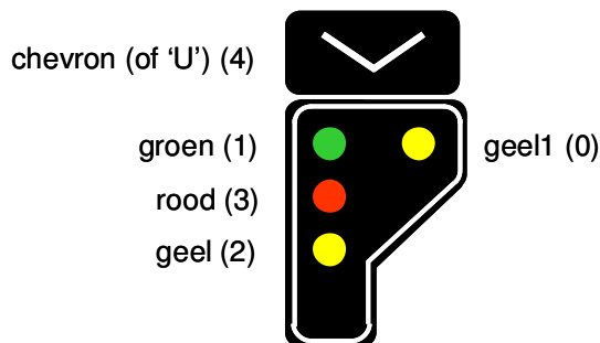
[5]BE: Bloksein met keper/U z wit
