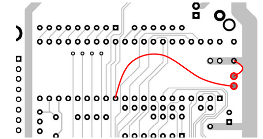
Fig 4: Extra verbindingen op PM32 voor bootloader
