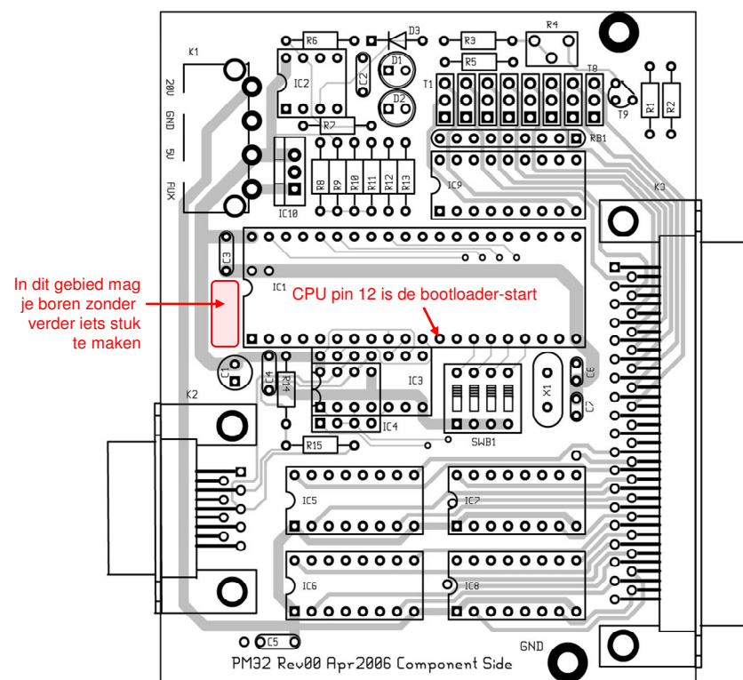
Fig 2: PM32 bovenaanzicht
