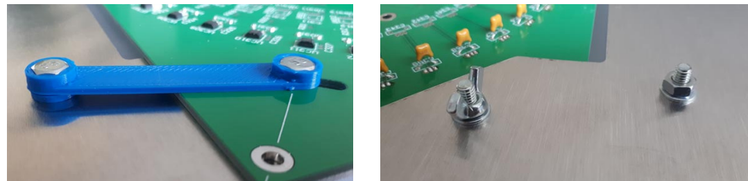
Abbildung 4: Verwendung Verriegelungsplatte
