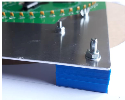
Abbildung 10: DTS montiert
