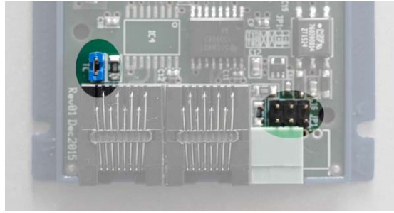
Fig 9: Jumper settings voor RM-C/1+ als RJ45↔wire-end tussenstation
