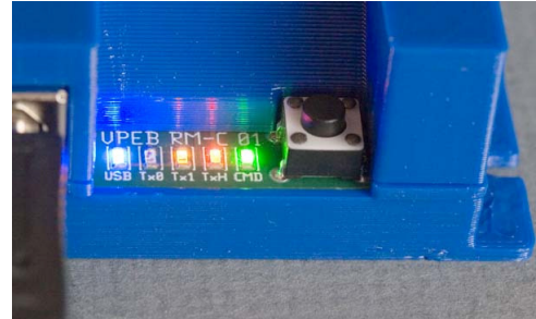
Fig 19: RM-C Reset knop naast de LEDs
