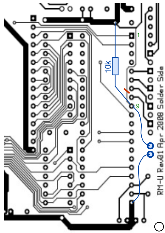
Fig 17: Aanpassingen RM-U Rev01/00 t.b.v. Reset-aansluiting
