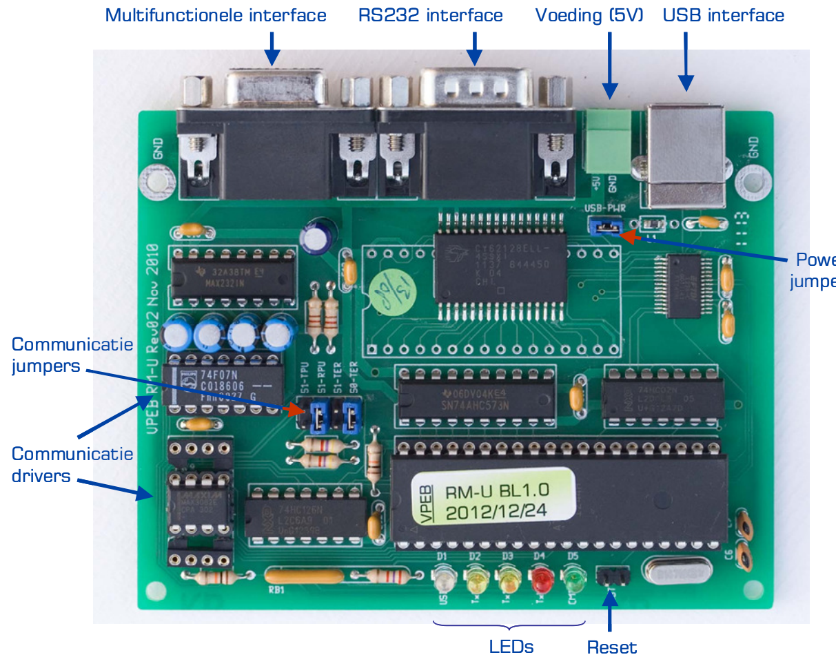
Fig 2: Opbouw en functies RM-U
